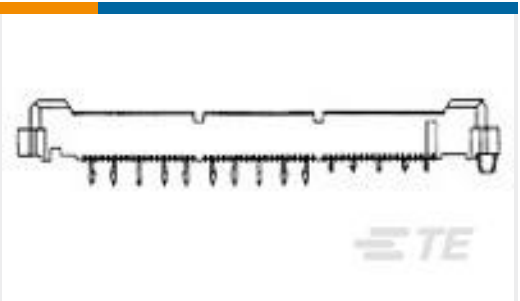
TE Part # 767153-8 38 POS. .355 VERTICLE RECEPTAC
